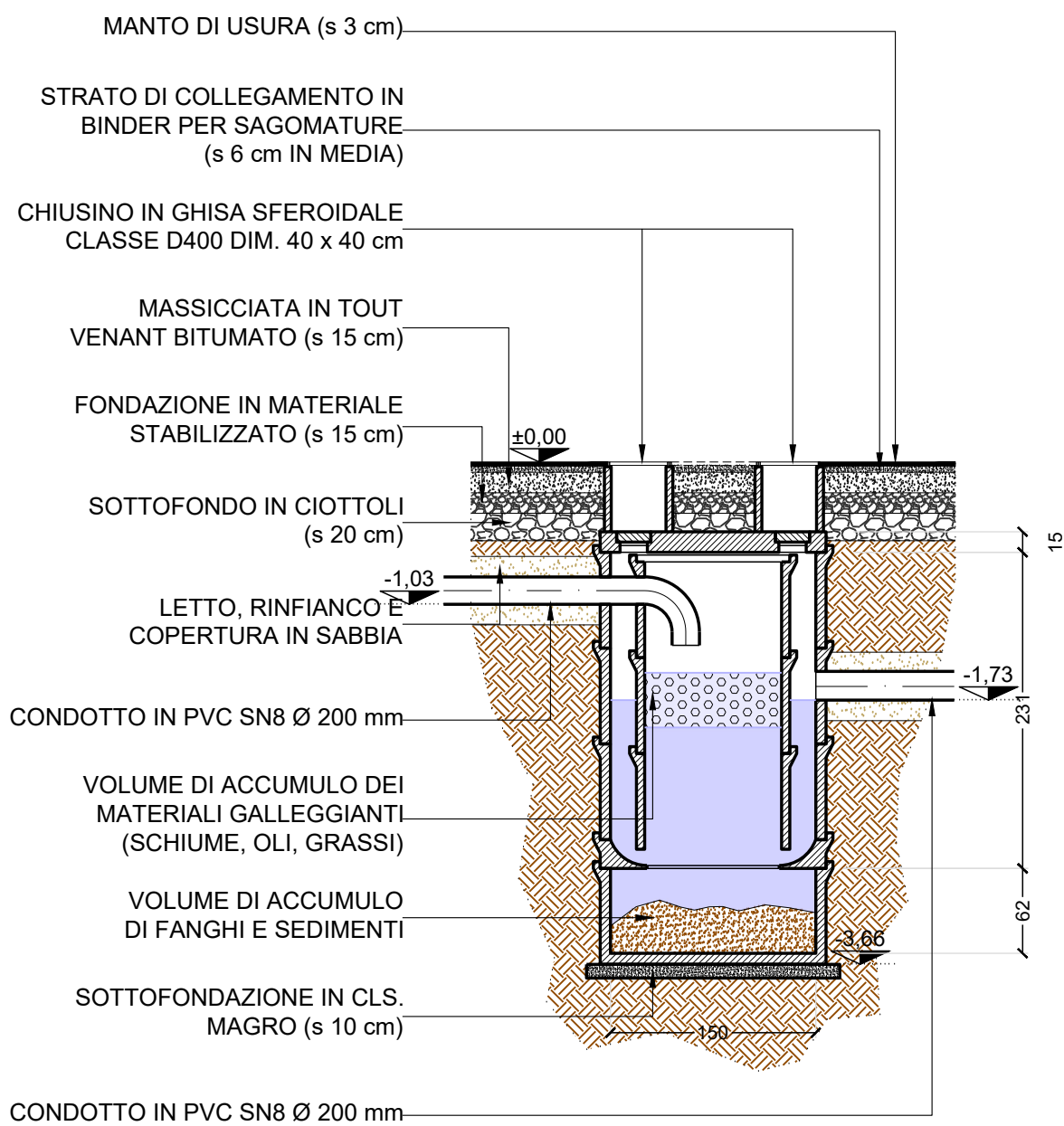
DISOLEATORE SEZIONE
