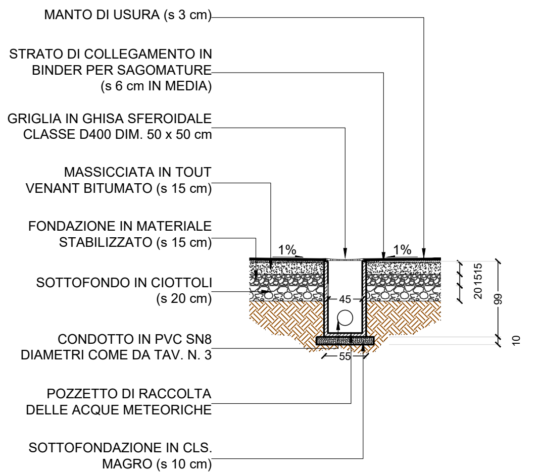
POZZETTO DI RACCOLTA DELLE ACQUE METEORICHE - SEZIONE
