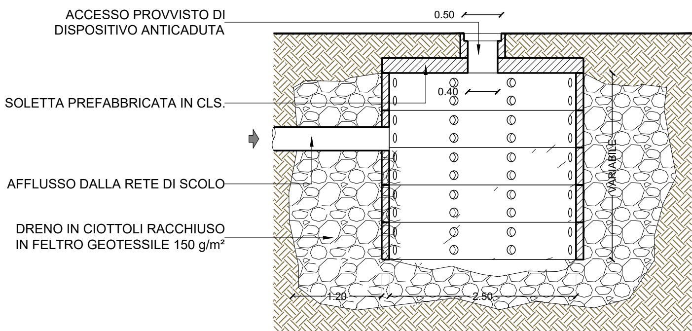
POZZO DISPERDENTE SEZIONE TIPO
