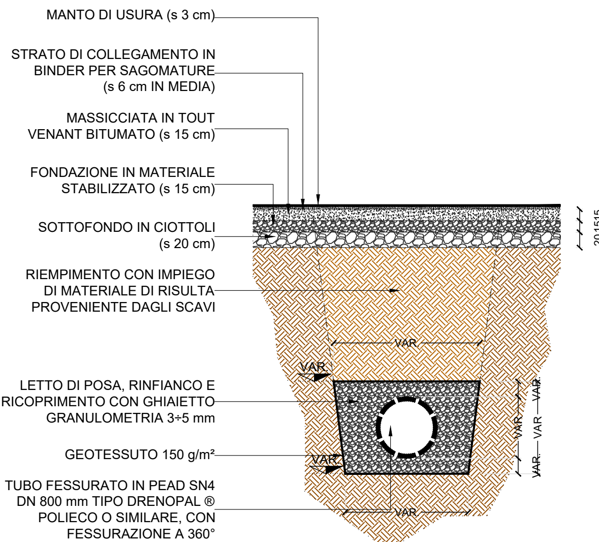
TRINCEA DI DISPERSIONE SEZIONE TIPO
