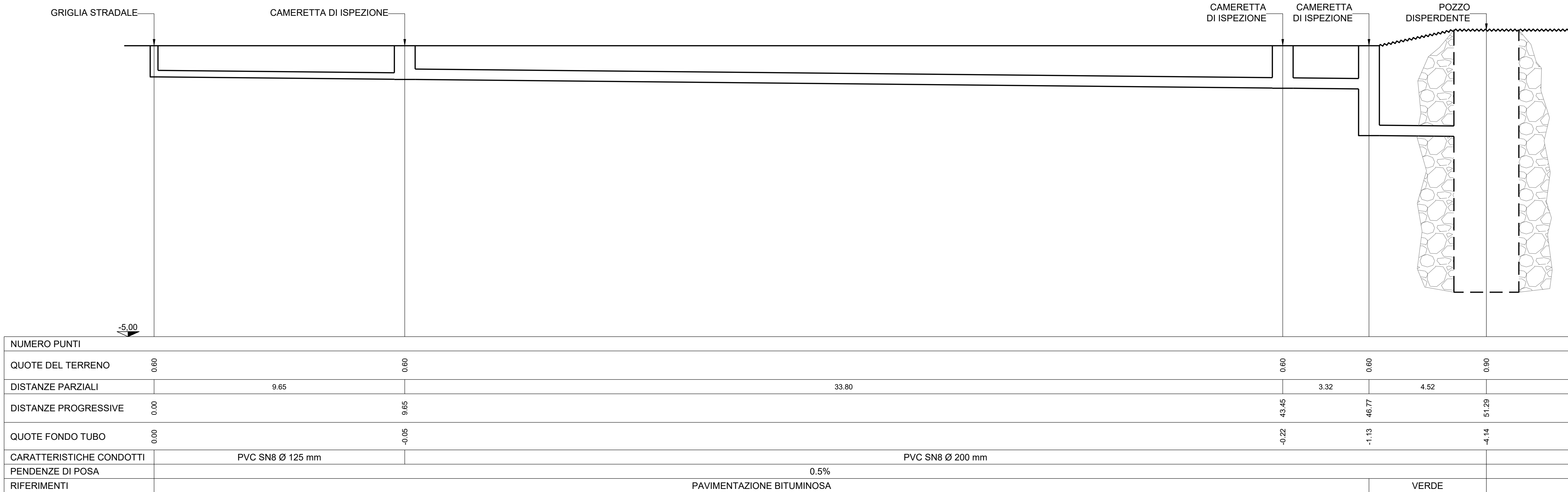
PROFILO DELLA LINEA DI RACCOLTA DELLE ACQUE DI DRENAGGIO METEORICO ASSERVITA AL NUOVO PARCHEGGIO DI VIA BIDINO - SCALA 1:50/1:100
