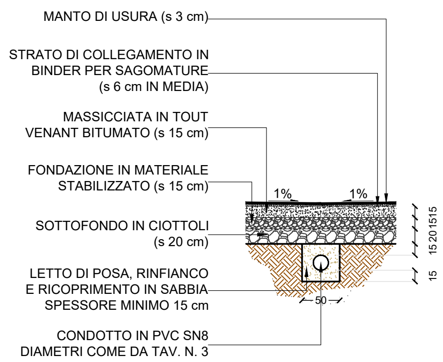
LINEA DI RACCOLTA DELLE ACQUE METEORICHE - SEZIONE TIPO
