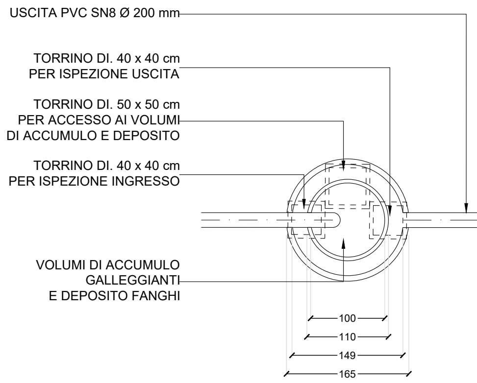
DISOLEATORE PIANTA
