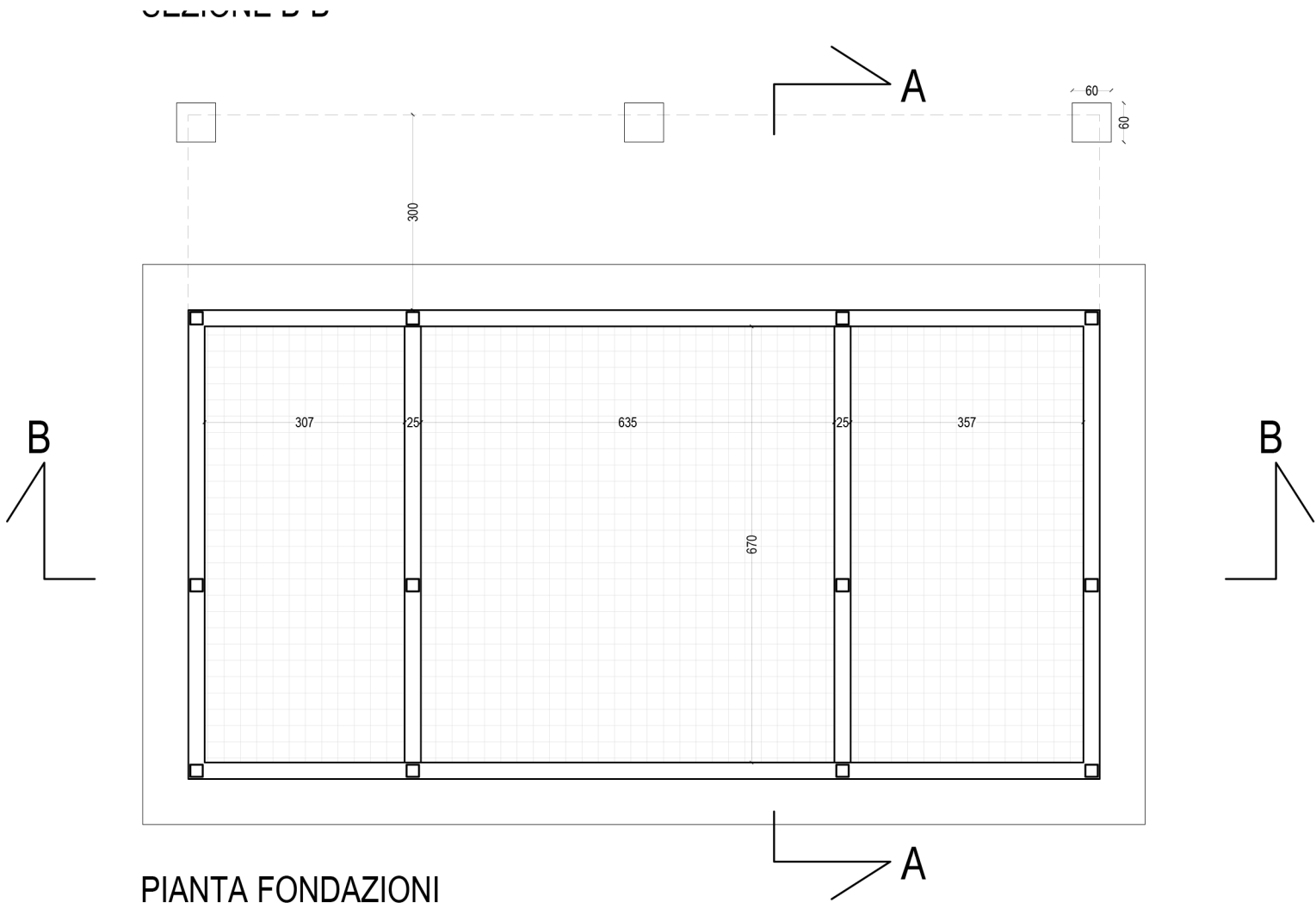
PIANTA FONDAZIONI
