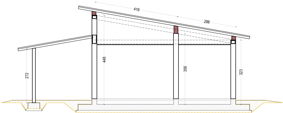
SEZIONE A-A
