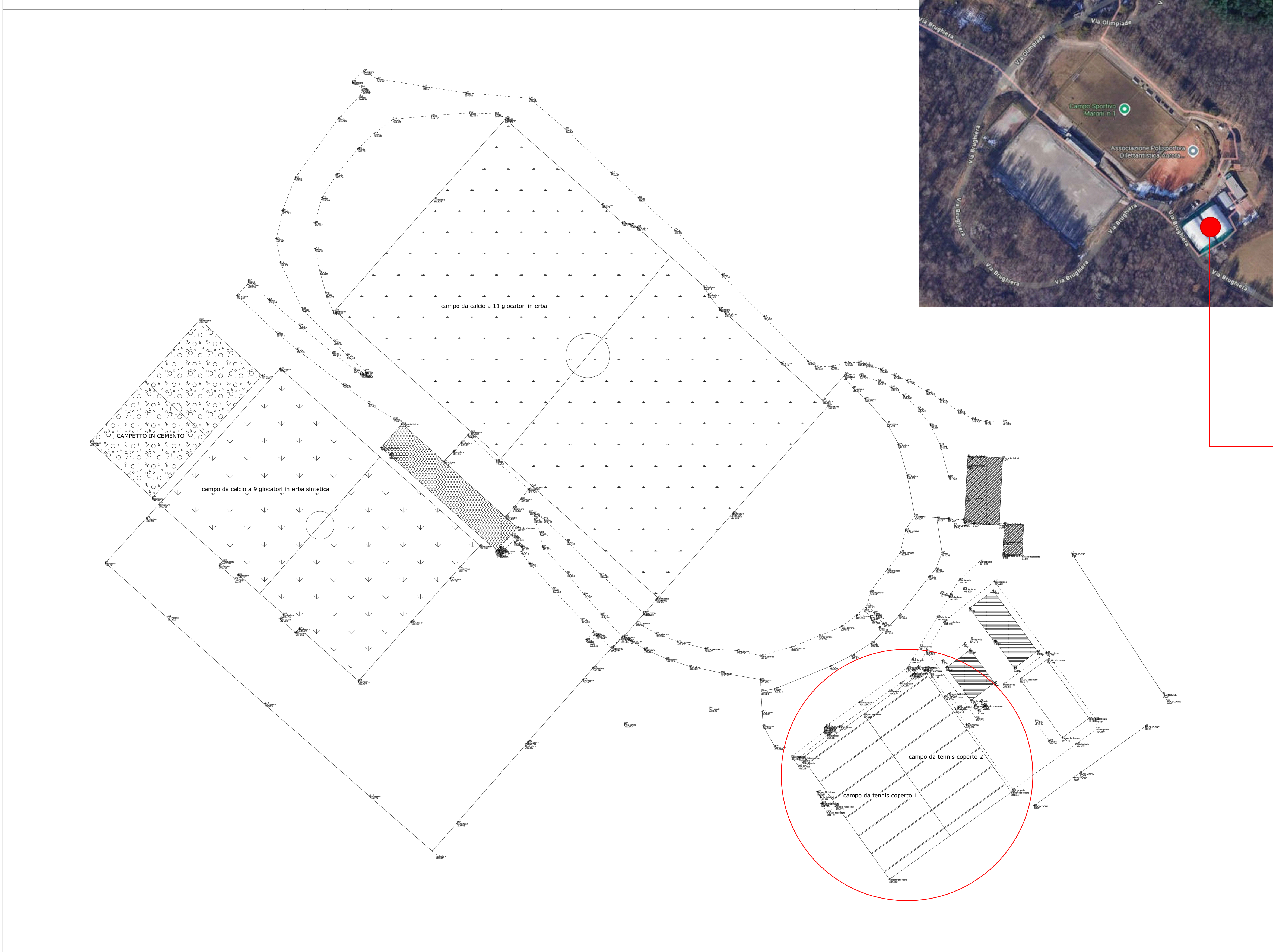
RILIEVO STATO DI FATTO – planimetria (scala 1:500)
