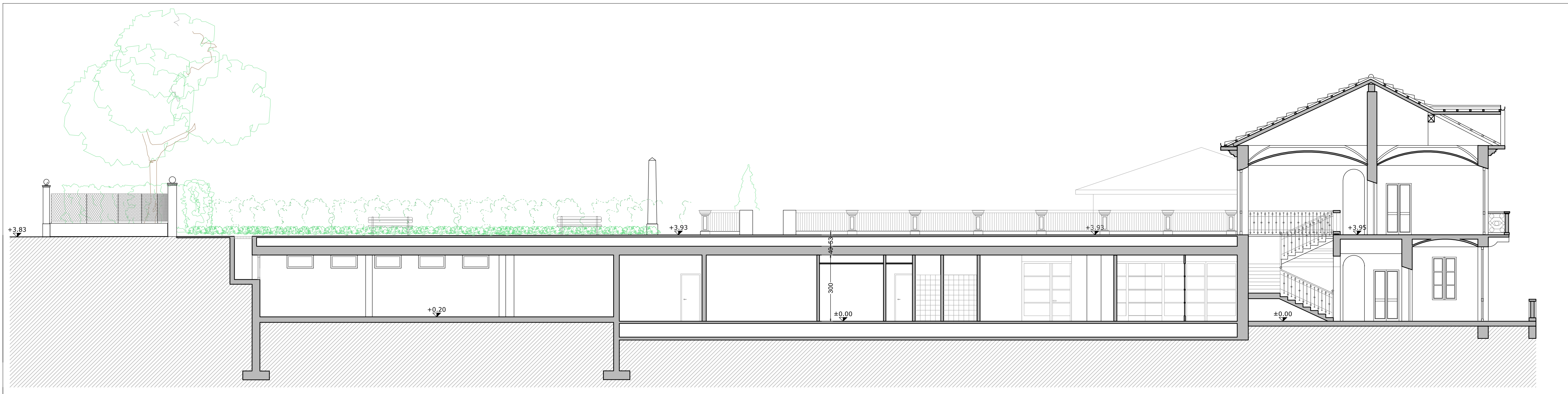
SEZIONE C-C
