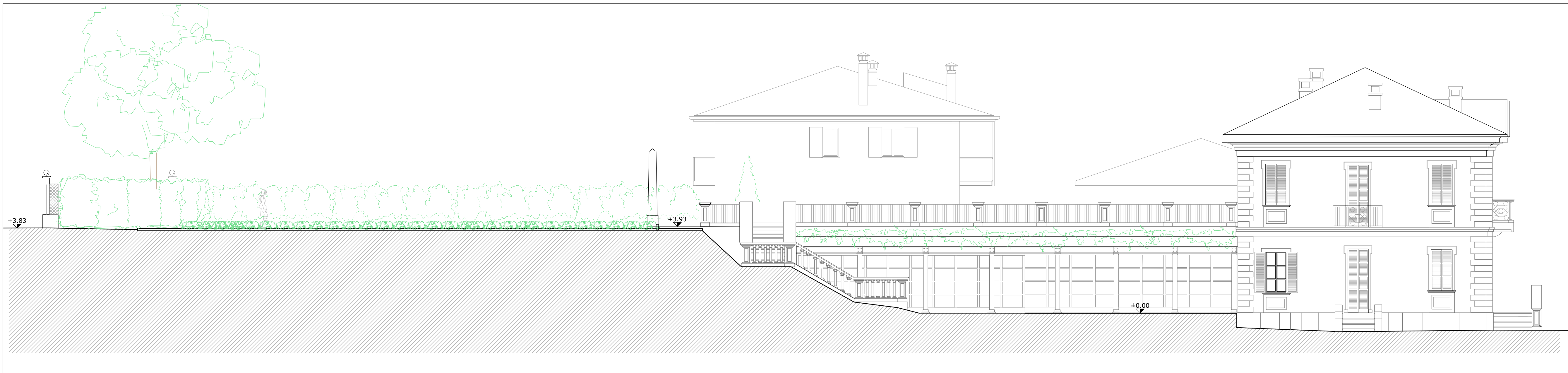
SEZIONE D-D
