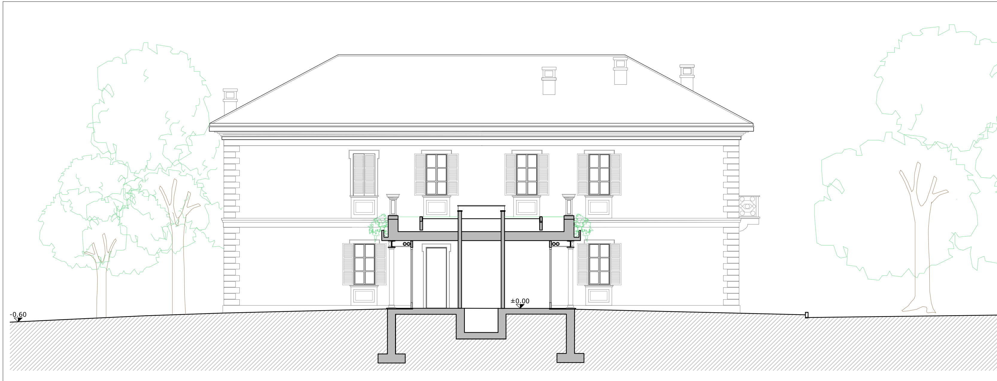
SEZIONE AA
