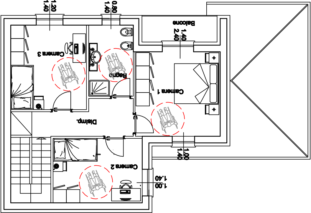
PIANO PRIMO
