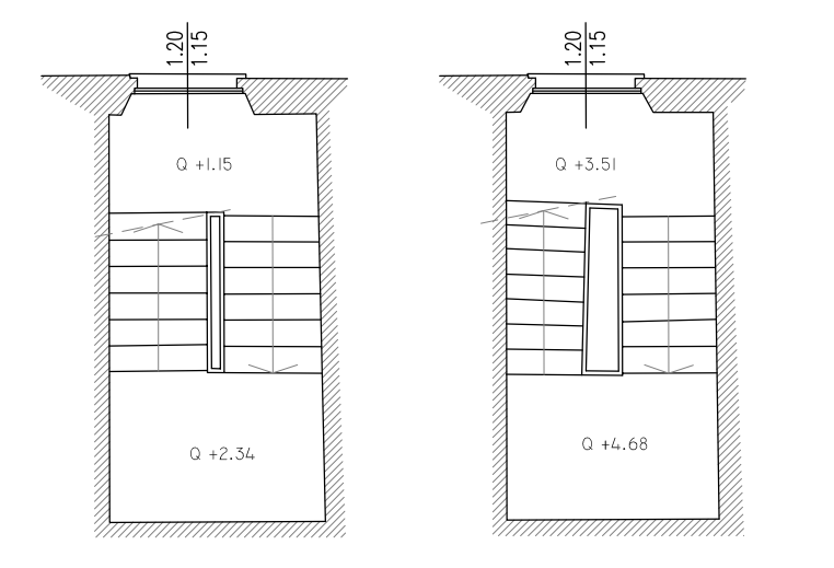
SCALA DAL PT AL P1/2 SCALA DAL P 1/2 AL P1
